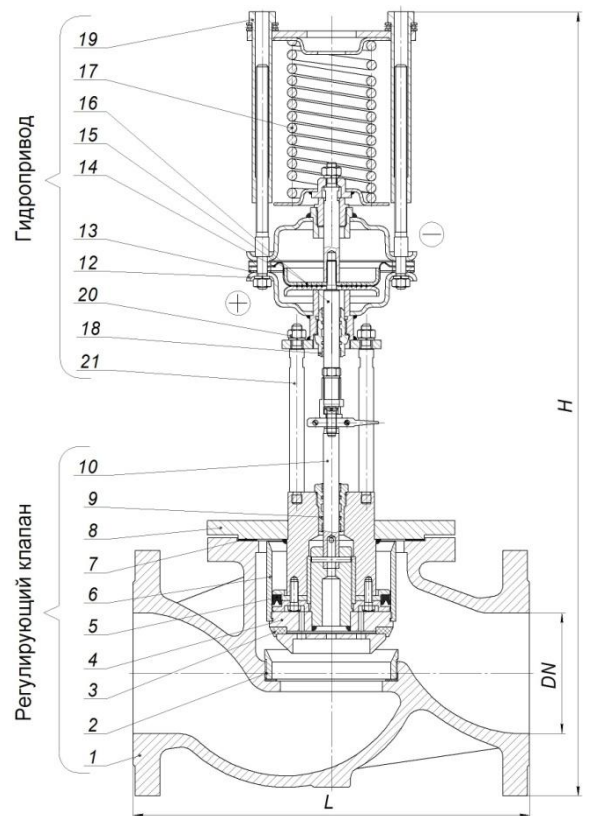
Рис.6 Регулятор УРРД-НЗ DN 125-300
