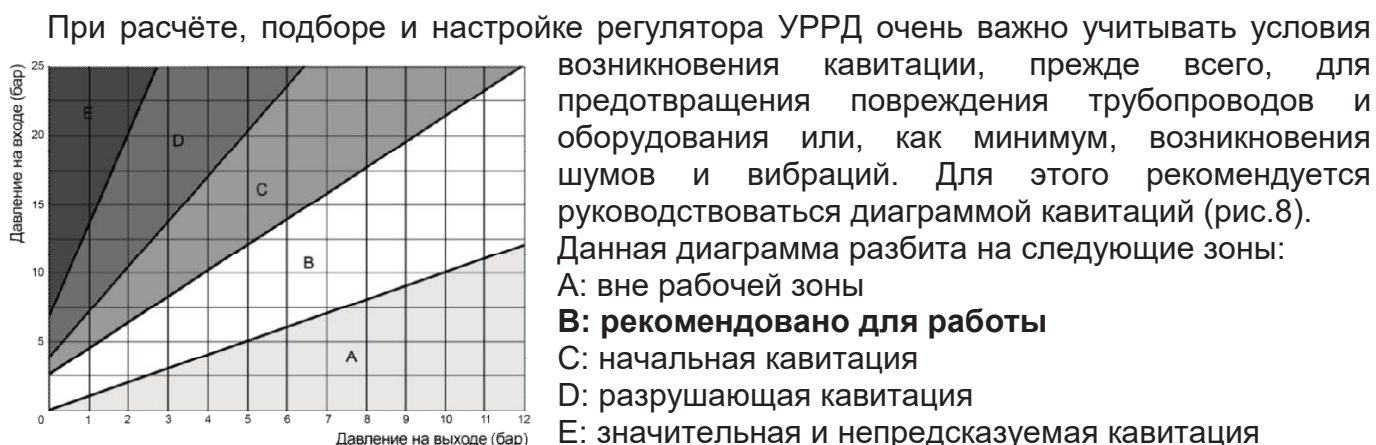
Рис.8 - Диаграмма кавитаций.
