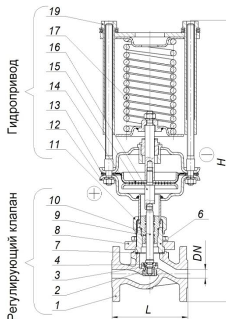
Рис.2 Регулятор УПРД–НЗ DN 15-32
