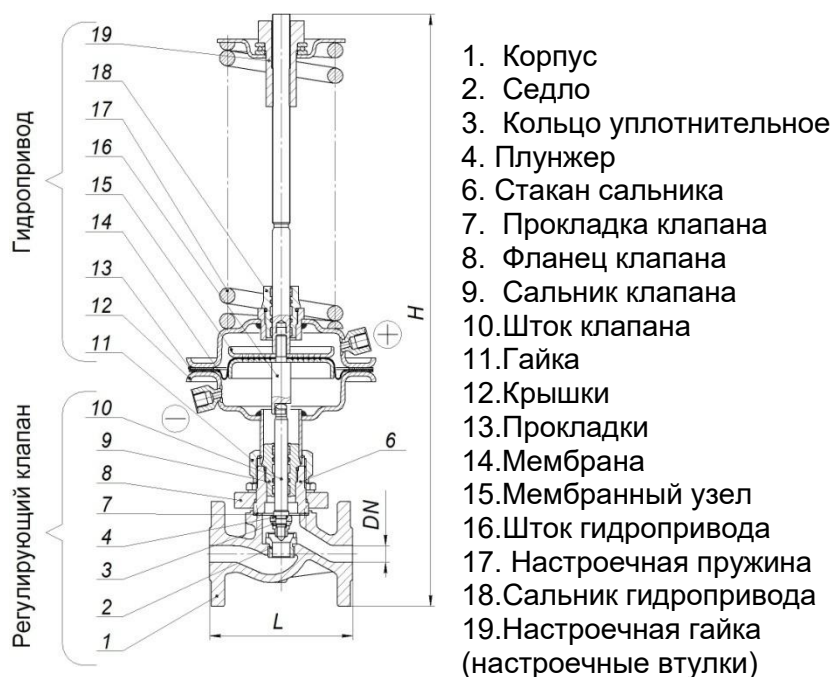
Рис.1 Регулятор УПРД–НО DN15-32
