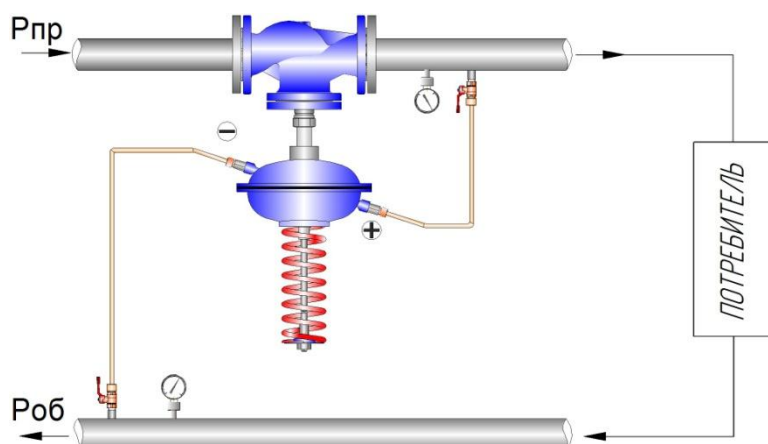
Рис.9 - Включение регулятора УРРД-НО «после себя»
