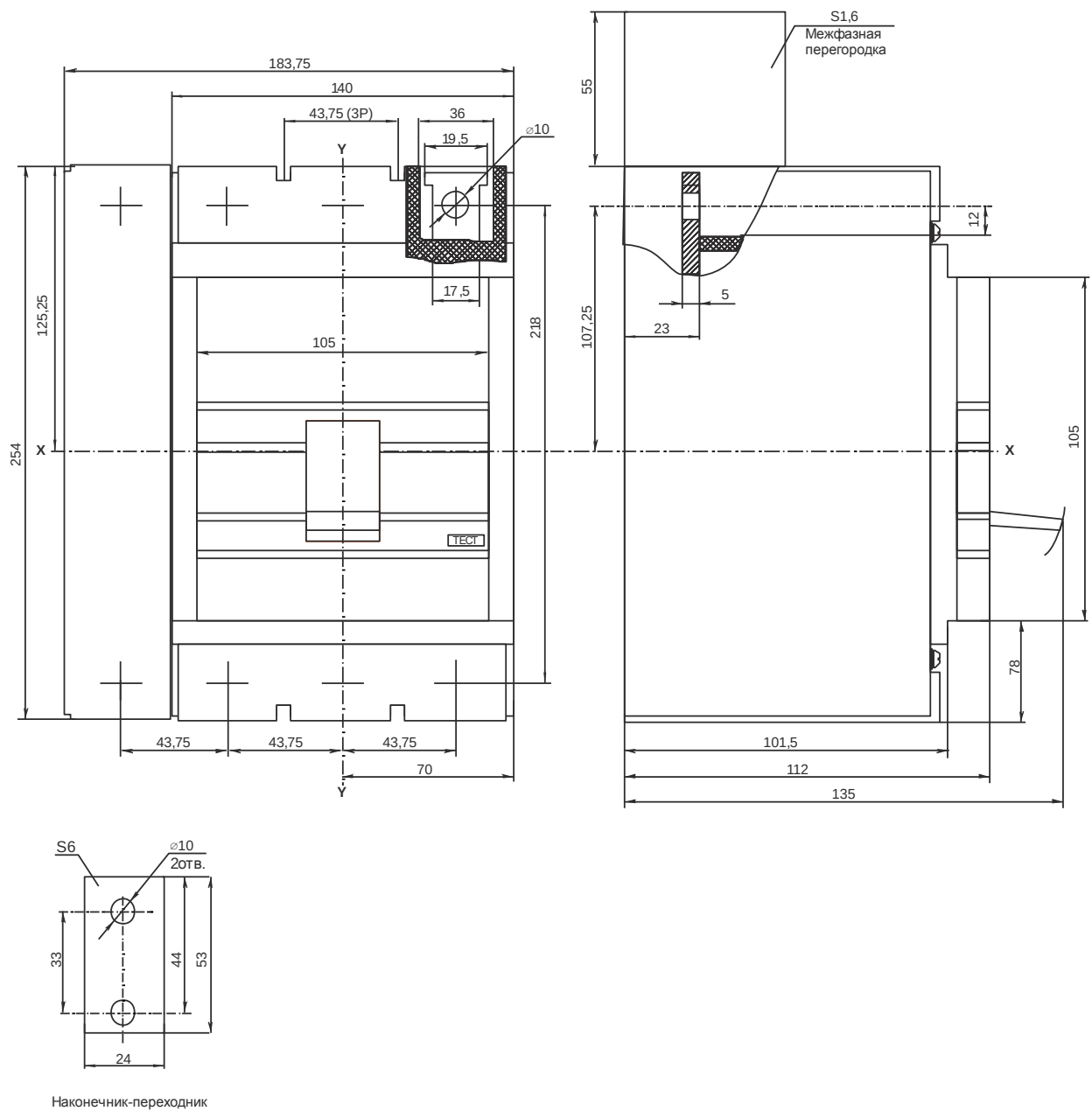
Рисунок 8 - Габаритные и установочные размеры выключателя ВА88-37
