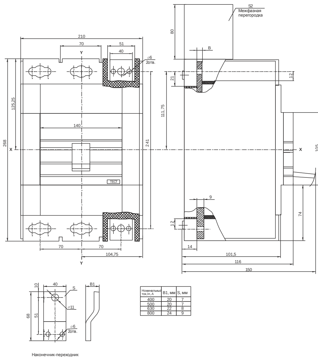
Рисунок 9 - Габаритные и установочные размеры выключателя BA88-40
