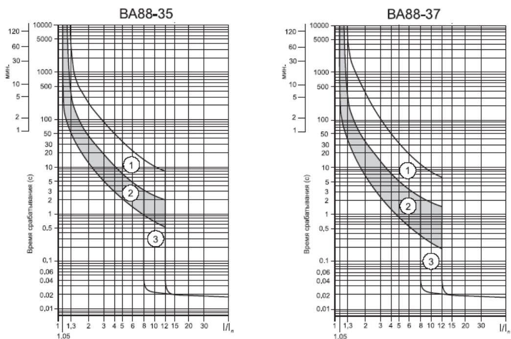
Рисунок 2 — Времятоковые характеристики выключателей BA88-35 и BA-37
