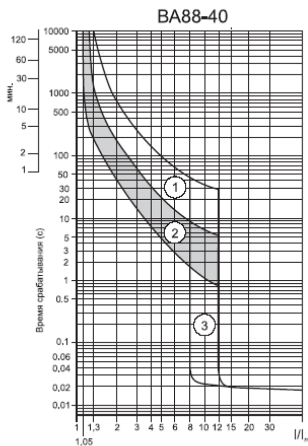
Рисунок 3 — Времятоковые характеристики выключателя BA88-40
