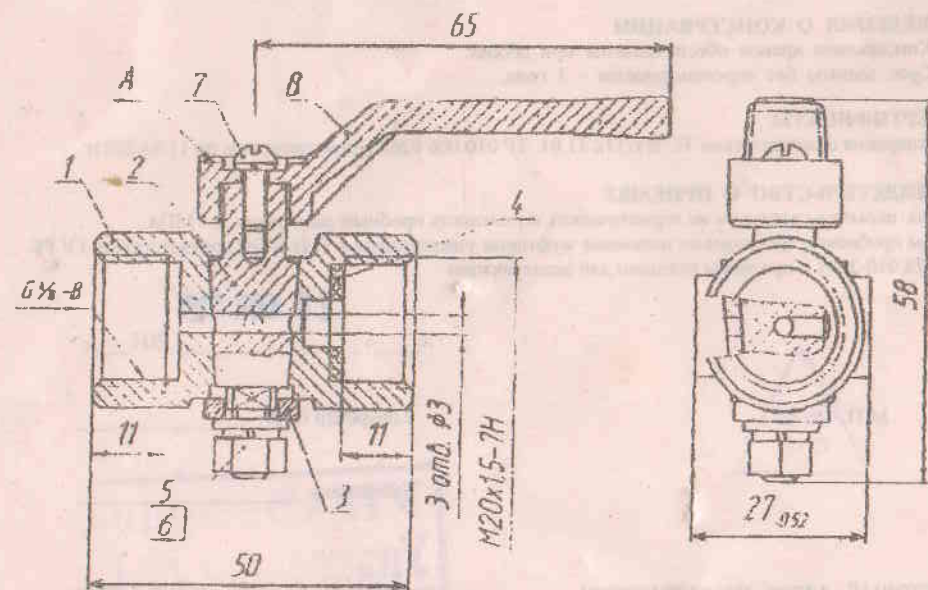
Рис. 3 – Кран КПТ 3.04.00
