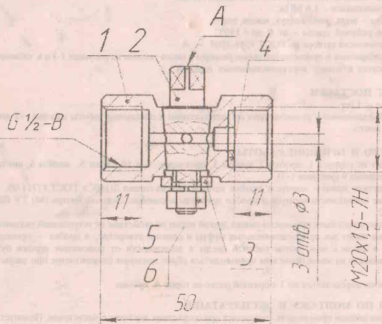
Рис. 1 – Кран КПТ 3.00.00
